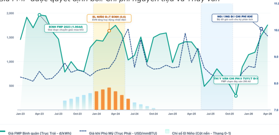
Hình: Phân Tích Tương Quan FMP: Thủy Văn vs. Giá khí Giá FMP được quyết định bởi: Chi phí nguyên liệu và Thủy văn
